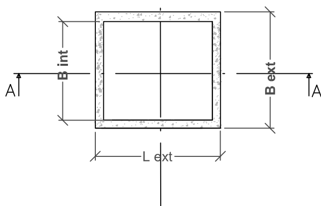
Doorsnede A-A / Coupe A-A
